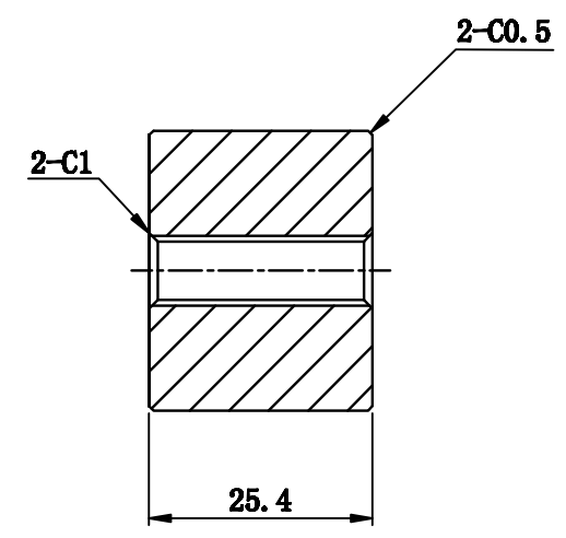
A-A
